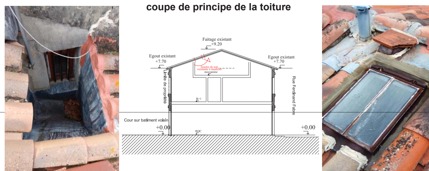
Vues sur les Velux existants à remplacer par fenetres "patrimoine" 80/120 sens de la pente pour le plus long coté, chevretres à reprendre pour les 4 faces coté rue Ferdinand Fabre coté cour interieure voisine
