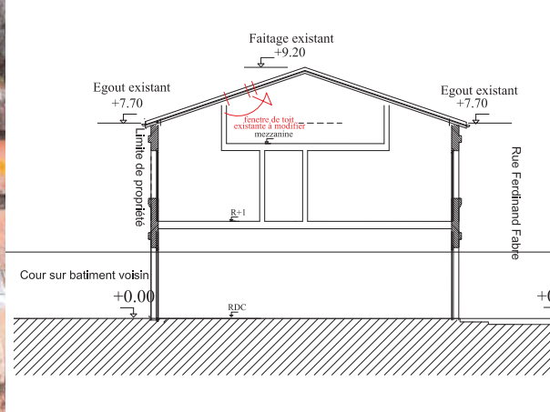
Vues sur les Velux existants à remplacer par fenestres "patrimoine" 80/120 sens de la pente pour le plus long coté, chevretres à reprendre pour les 4 faces coté rue Ferdinand Fabre coté cour interieure voisine
